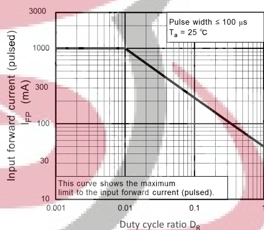
Fig. 12.4 I_{FP} - D_R
